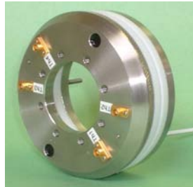
Projet Thermosavant 4-canal- Mesure de Temperature dans Centrifugeuse
